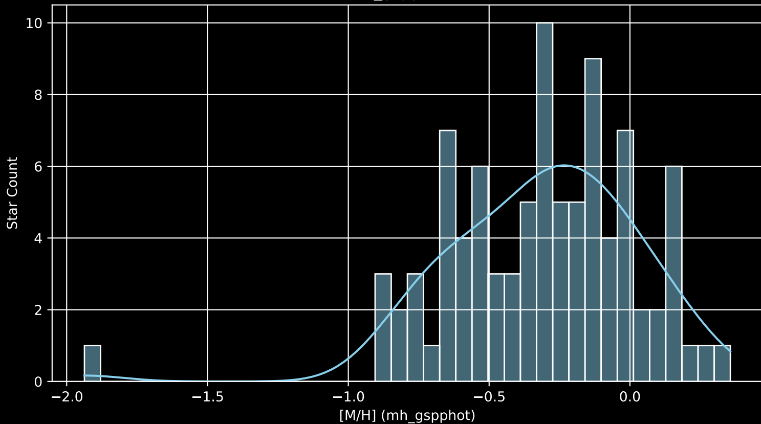
GALAH DR4 Field: [6683] [M/H] (mh_gspphot) (n= 91)
