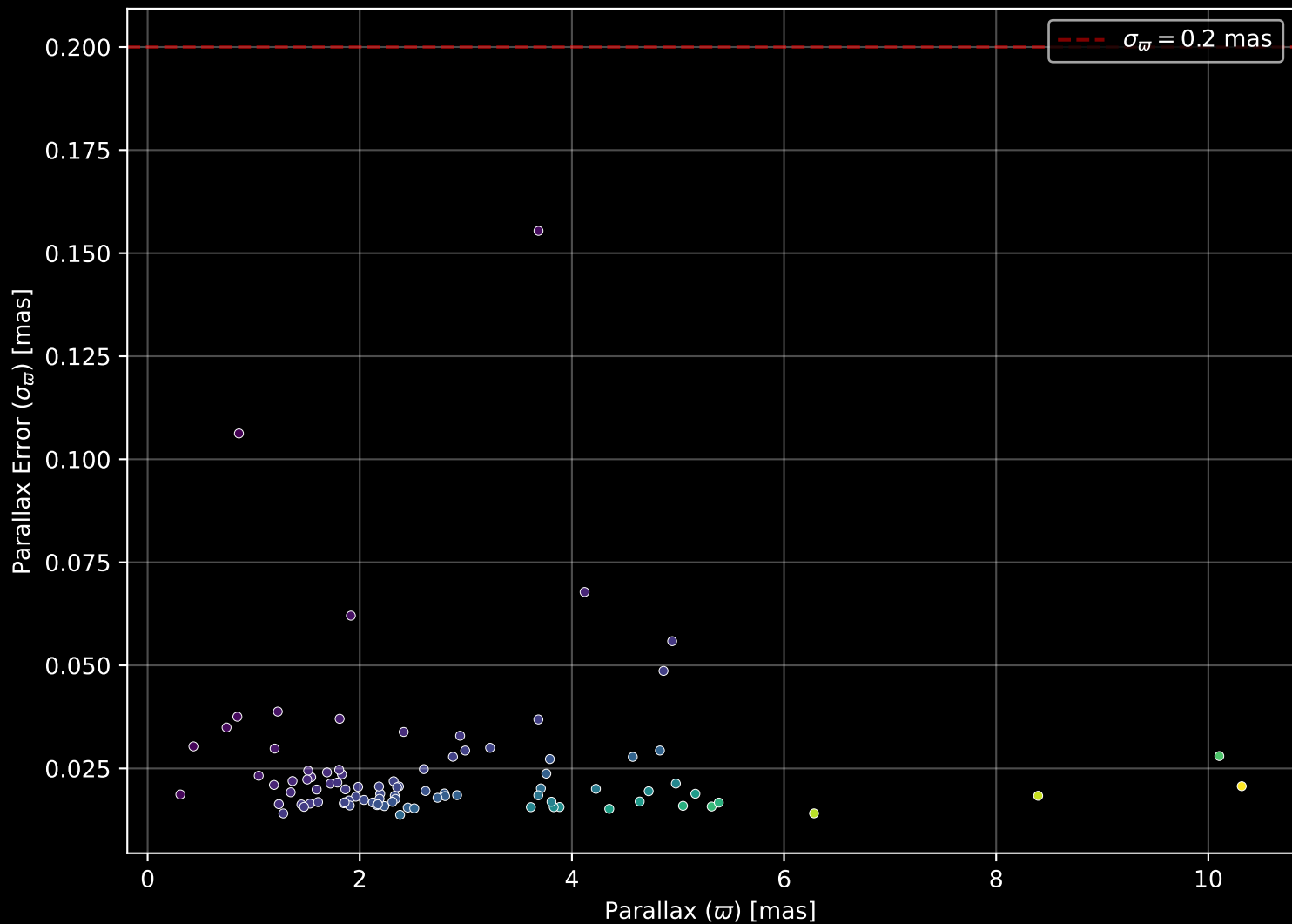
GALAH DR4 Field: [6683] Parallax Quality (n= 91)
