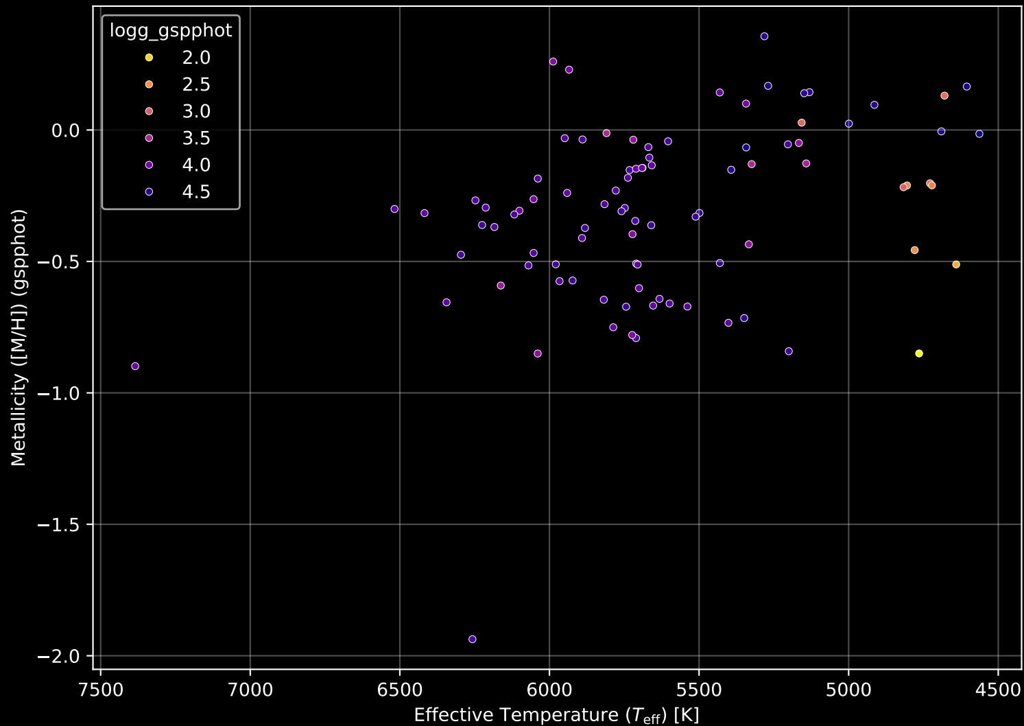
GALAH DR4 Field: [6683] Stellar Population Parameters (n= 91)
